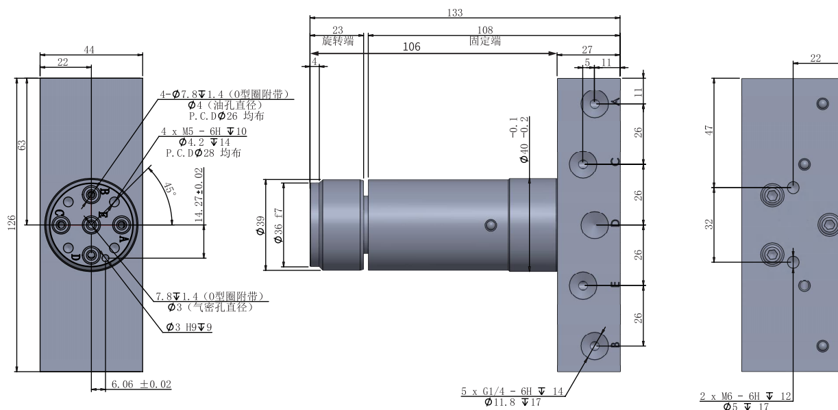
10960501 尺寸图:
