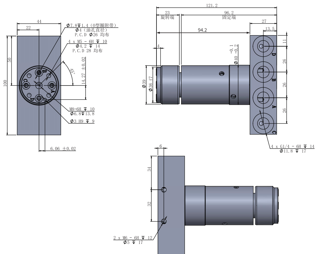
10960401 尺寸图:
