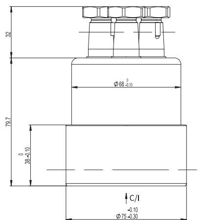
图示为油缸压紧状态 富余行程3mm
