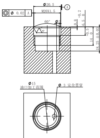
1106-FLS-20T 安装尺寸图
